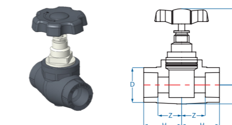
VAN XOAY / Gate valve
