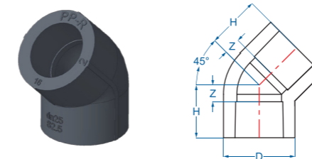
CO 45° / 45° Elbow
