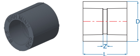
NỐI TRƠN / Plain socket
